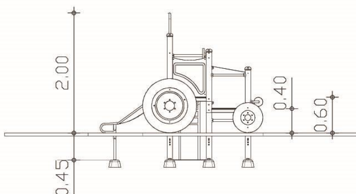
όψη
