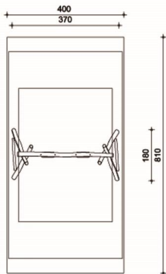
κάτοψη
