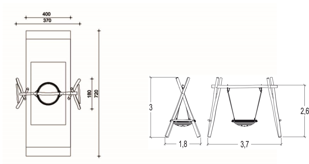
όψεις
