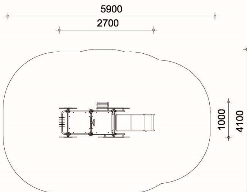
κάτοψη
