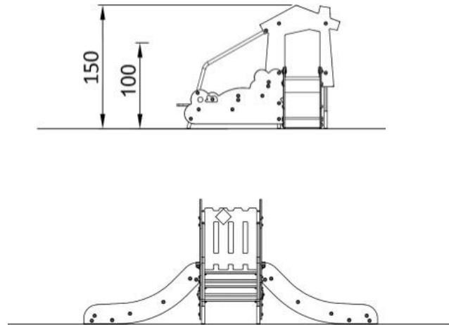
όψεις
