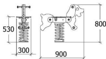
όψη
