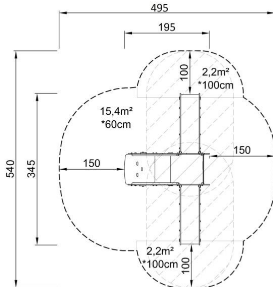
κάτοψη
