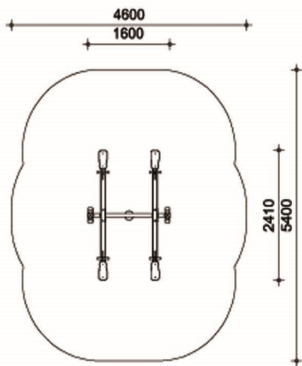
κάτοψη
